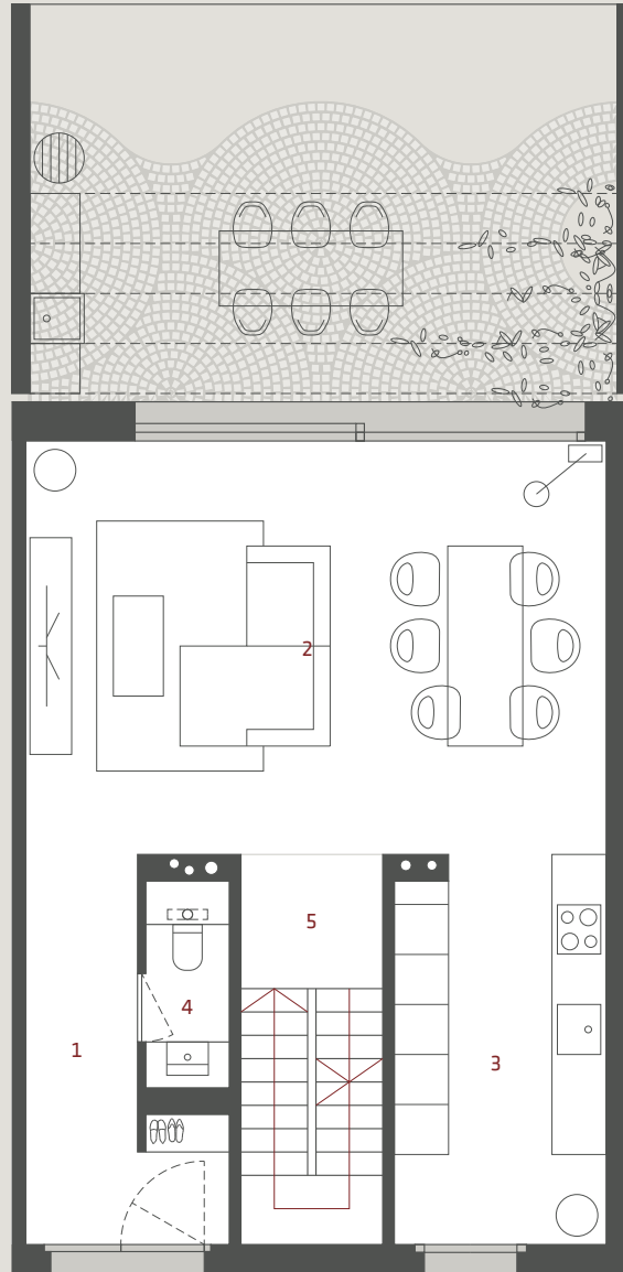
PRITLIČJE
