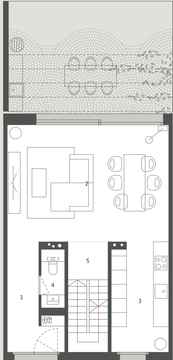
PRITLIČJE
