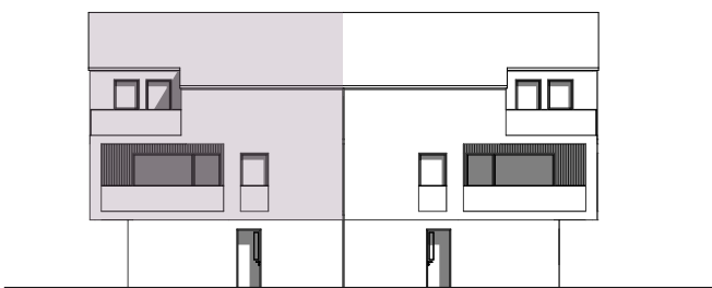
SEVEROZAHODNA FASADA
